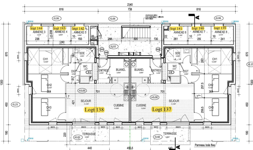
PLAN RDC 1/100
